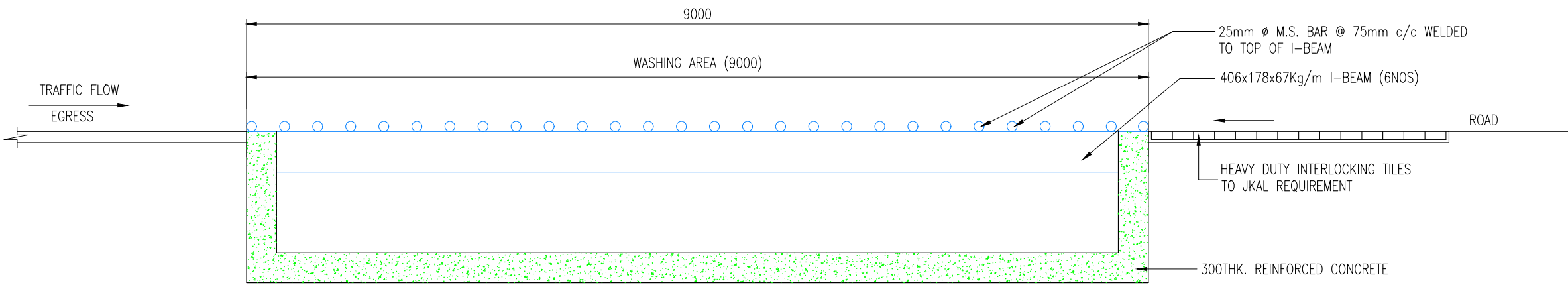
LONGITUDINAL SECTION (Y - Y) SCALE 1:50
