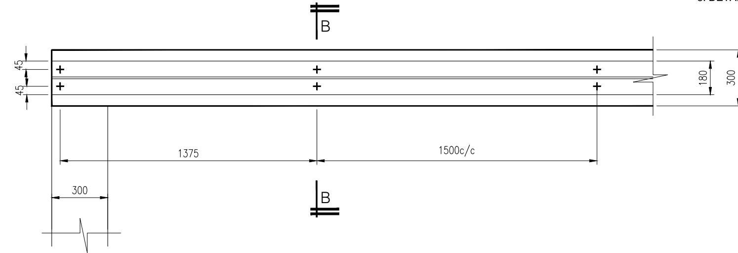
DETAIL '2' SCALE : 1:20
